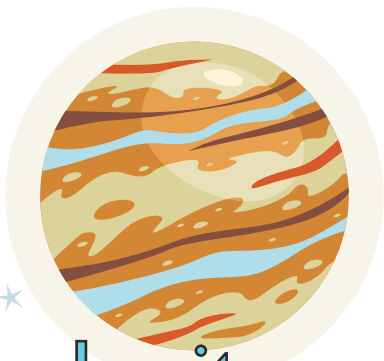
Jupiter
